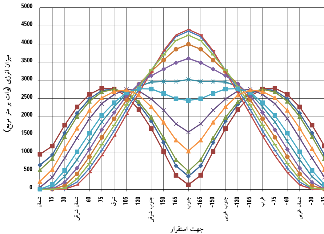
انرژی خورشیدی تابیده شده بر سطوح عمودی در عرض جغرافیایی 26 درجه شمالی
