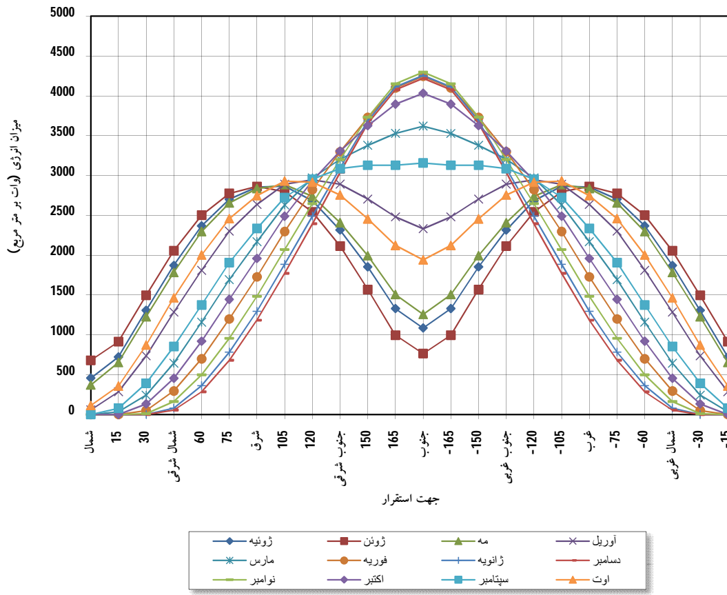
انرژی خورشیدی تابیده شده بر سطوح عمودی در عرض جغرافیایی 34 درجه شمالی
