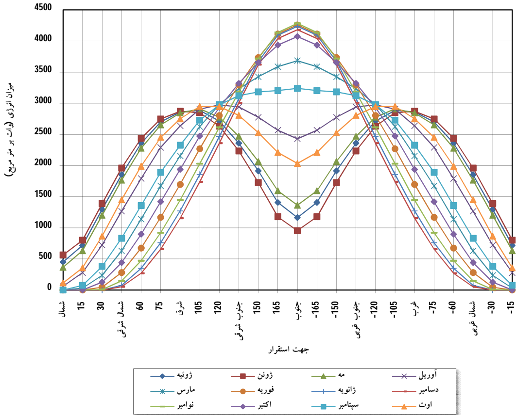
انرژی خورشیدی تابیده شده بر سطوح عمودی در عرض جغرافیایی 35 درجه شمالی
