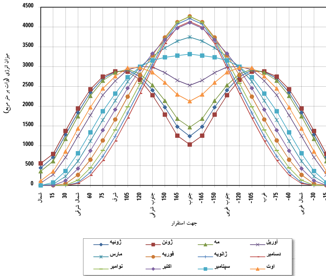
انرژی خورشیدی تابیده شده بر سطوح عمودی در عرض جغرافیایی 36 درجه شمالی
