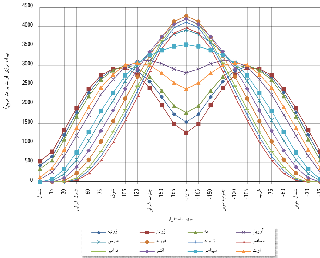
انرژی خورشیدی تابیده شده بر سطوح عمودی در عرض جغرافیایی 39 درجه شمالی
