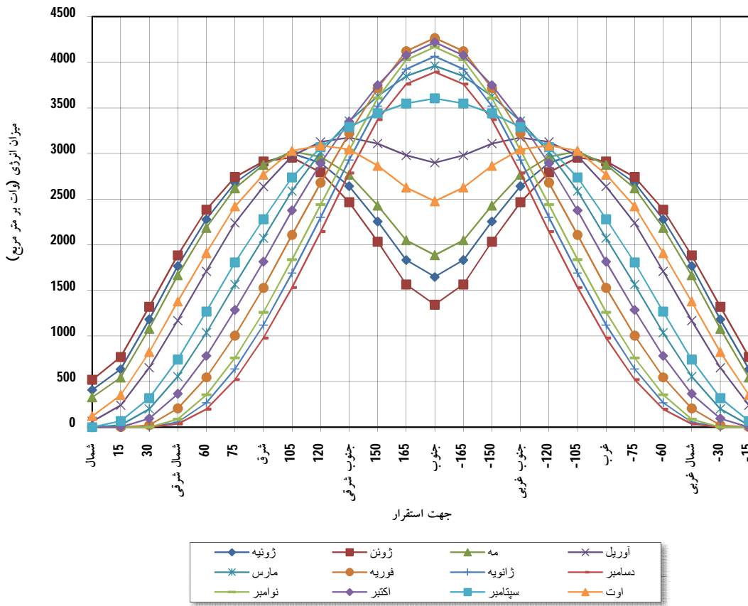
انرژی خورشیدی تابیده شده بر سطوح عمودی در عرض جغرافیایی 40 درجه شمالی
