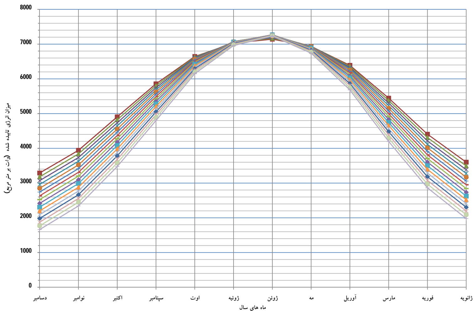
میزان انرژی خورشیدی تابیده شده بر سطوح افقی در اولین روز از هر ماه در عرض های جغرافیایی 25 تا 40 درجه شمالی
