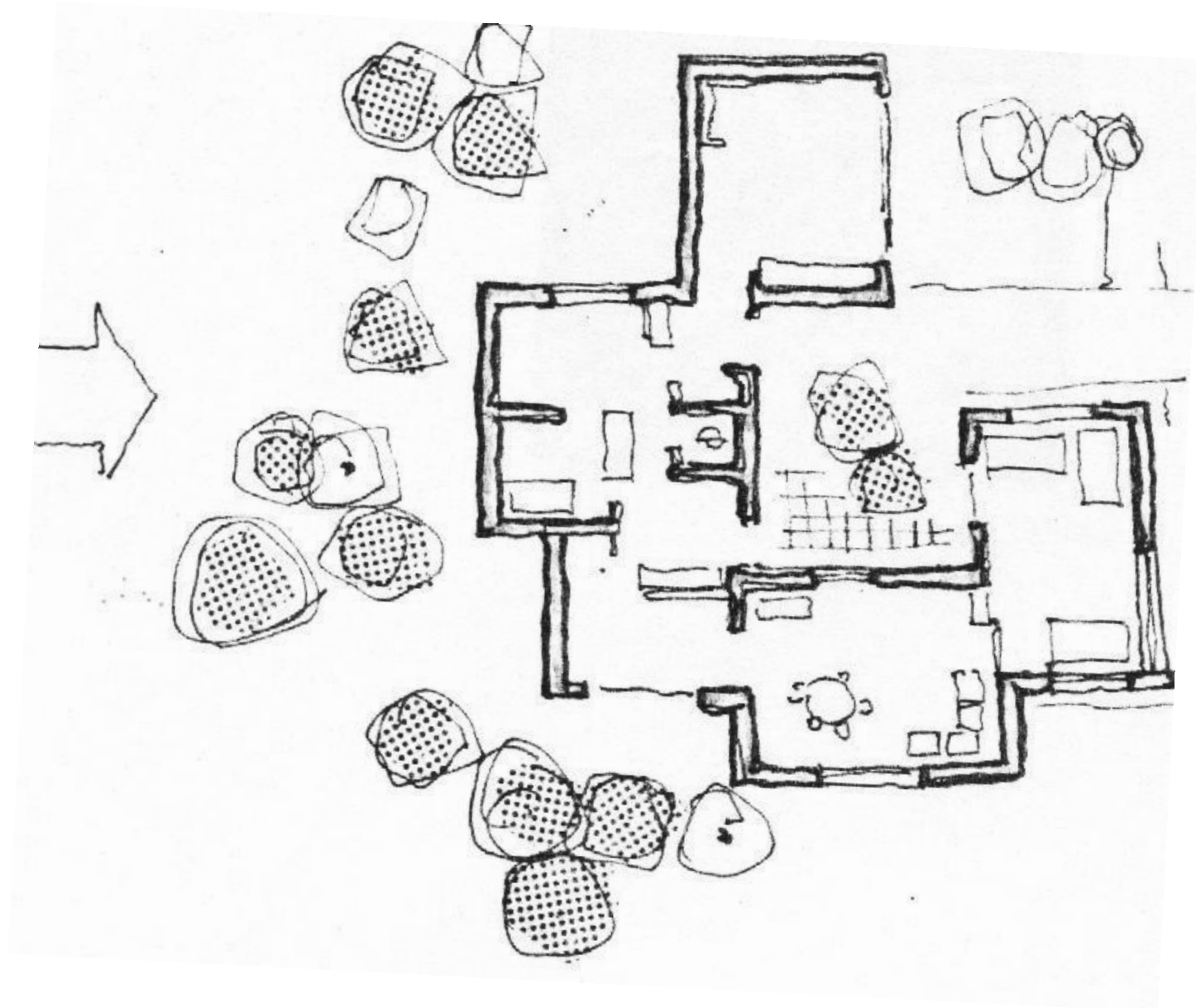
فاصله بین دیوارهای خارجی، بوته‌ها و شاخ و برگ درختان امکان بازتاب حرارت از دیوارهای خارجی و خنک سازی آنها را فراهم می‌سازد (طرح از محمد خسروشاهی).
