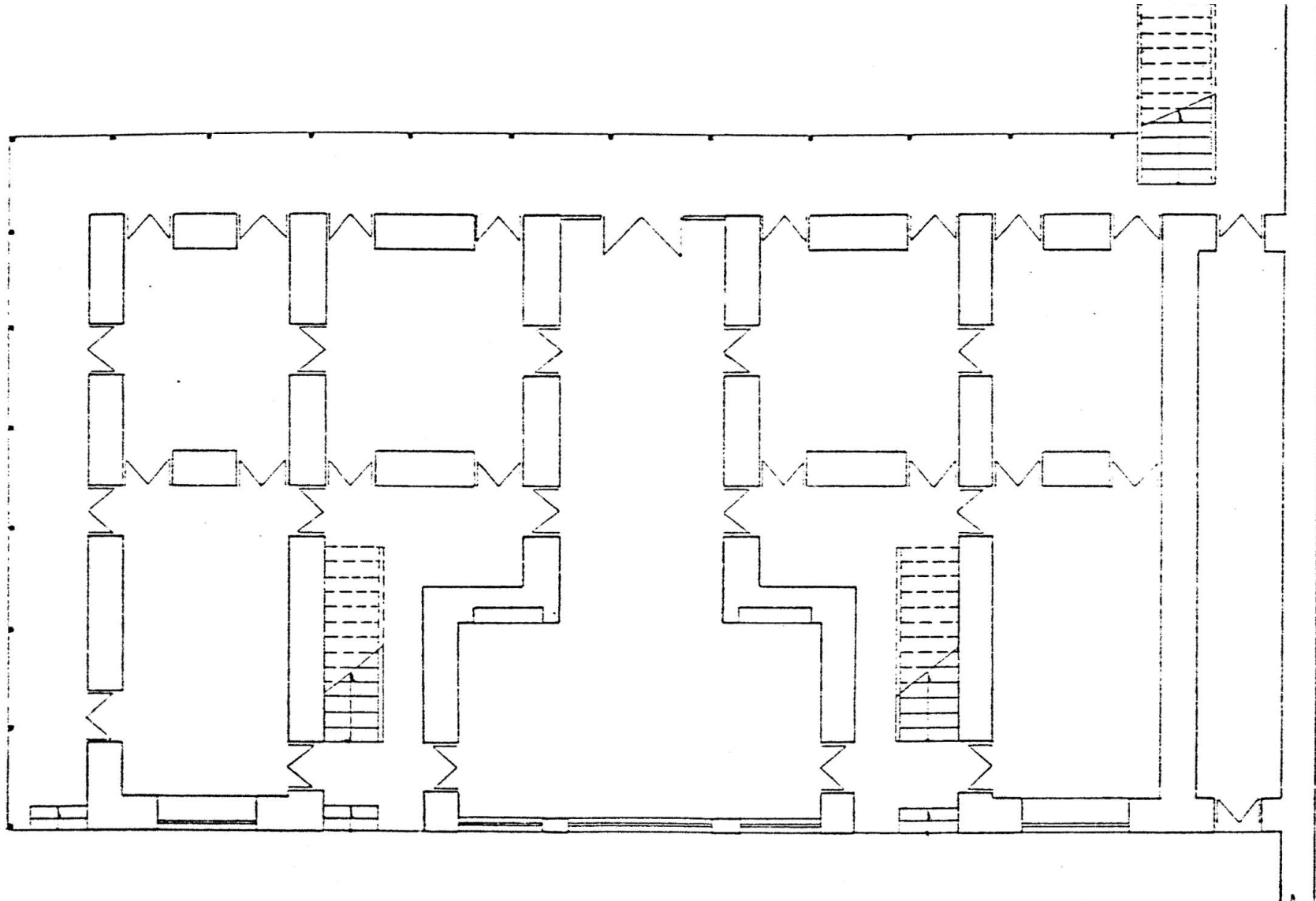
تعییه درهای ارتباطی بین اتاقها امکان هدایت جریان هوا به همه اتاقها را فراهم می‌سازند (پلان طبقه همکف خانه ابریشمی در رشت)
